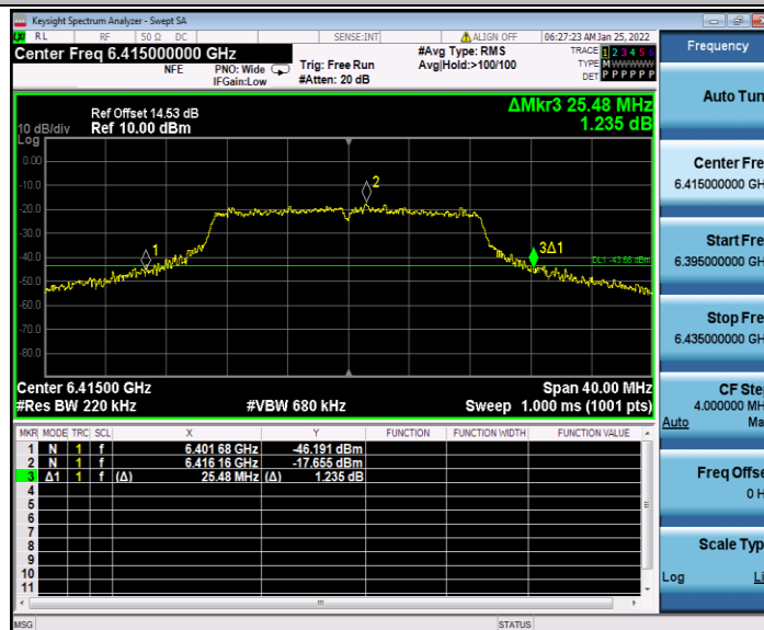
11N20MIMO_Ant2_6415
