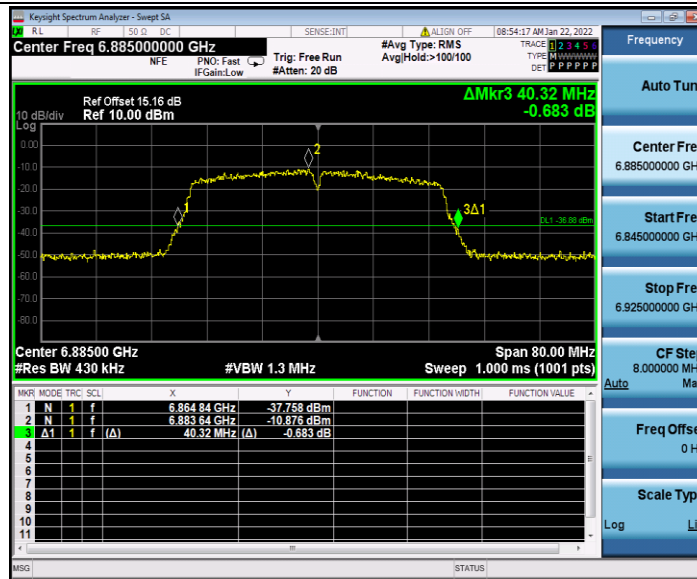
11N40SISO_Ant2_6885
