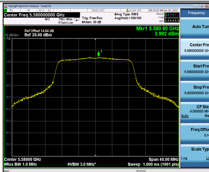
11AX20MIMO_Ant1_5580
