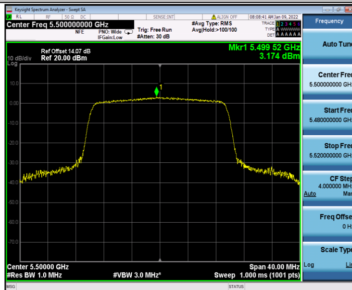
11AX20SISO_Ant2_5500
