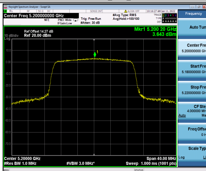
11AX20SISO_Ant2_5200
