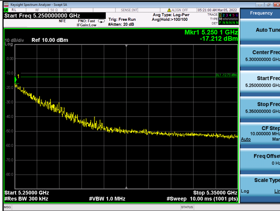
11n20 5240 Ant 2
