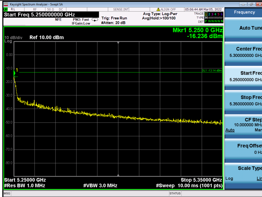
11n40 5230 Ant 2
