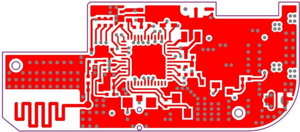
Top Layer
