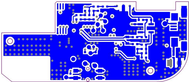
Bottom Layer
