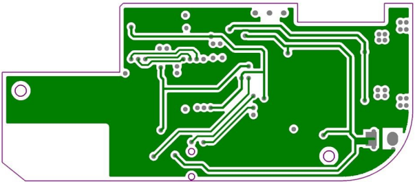
VCC Layer
