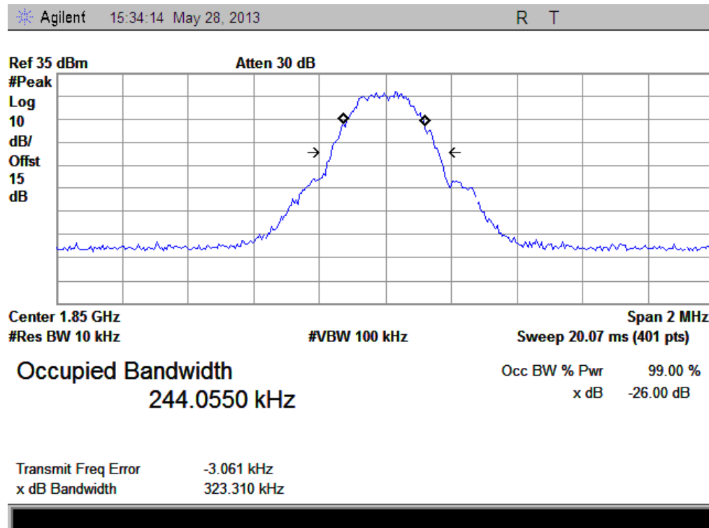
(Plot Q1: GPRS 1900MHz Channel = 512)
