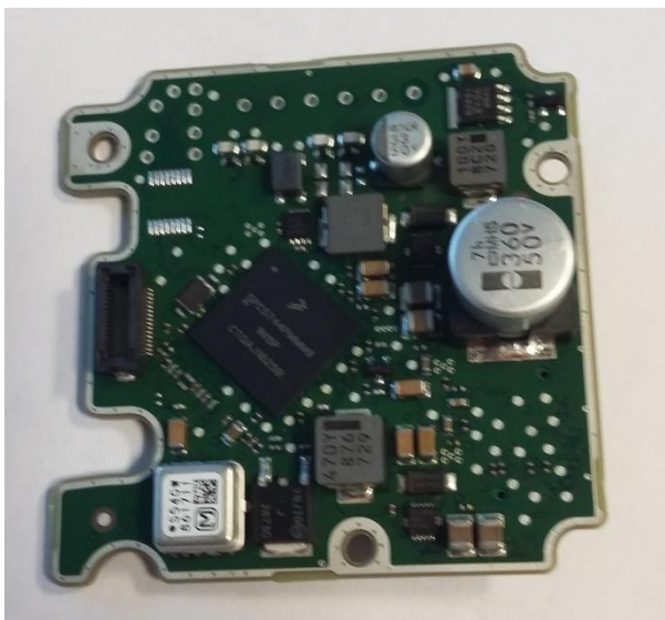
DSP PCB - Side 1
