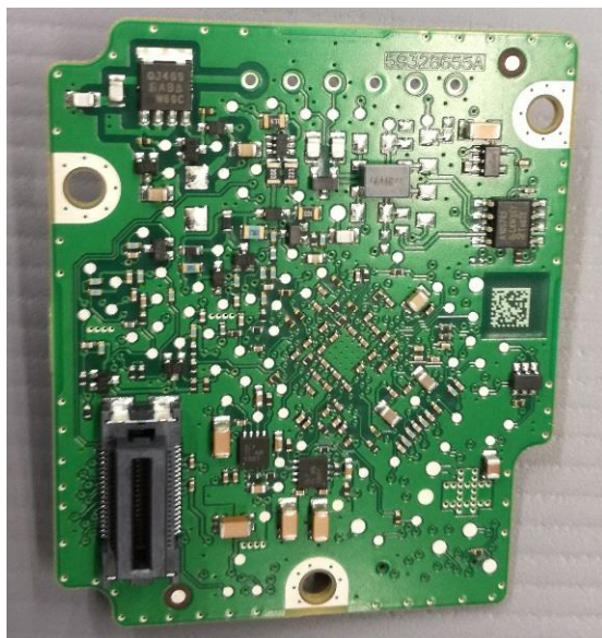
DSP PCB - Side 1
