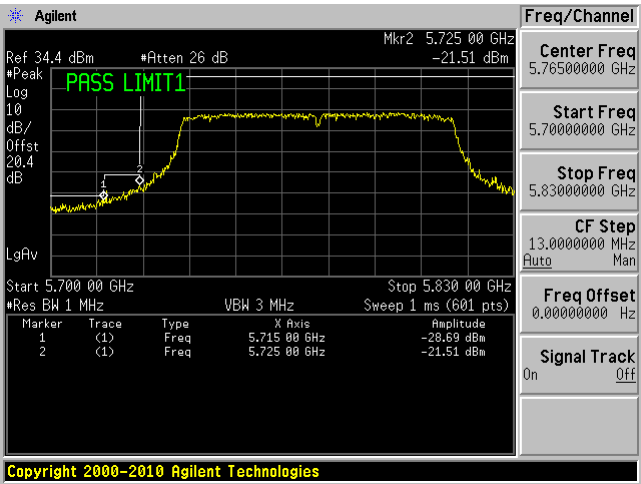
Chain 1 Lower Band Edge
