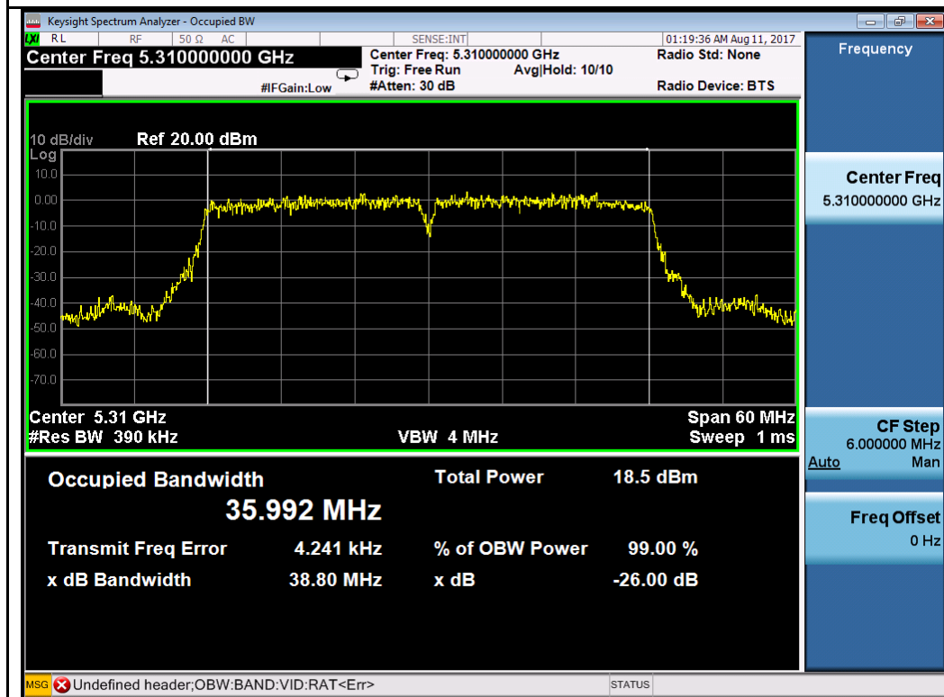
802.11n-HT40-5310MHz
