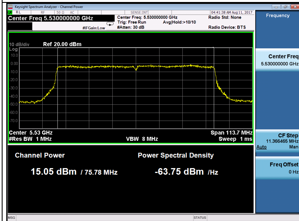
802.11ac-VHT80 5530M
