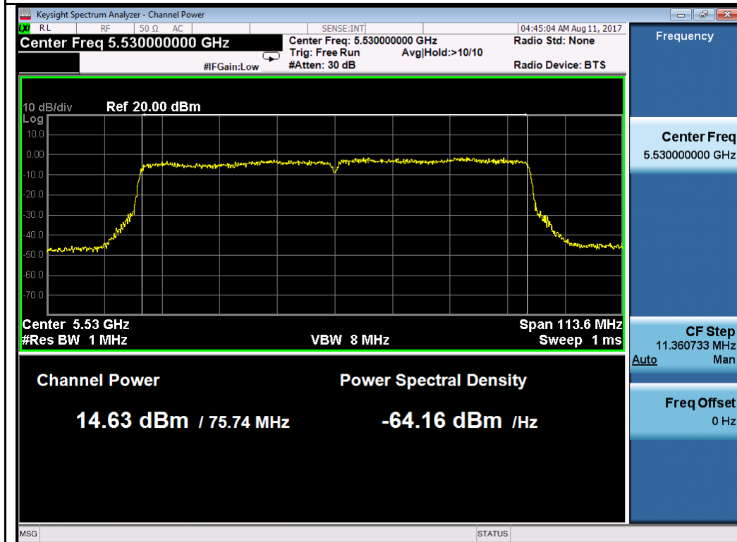
802.11ac-VHT80 5530M
