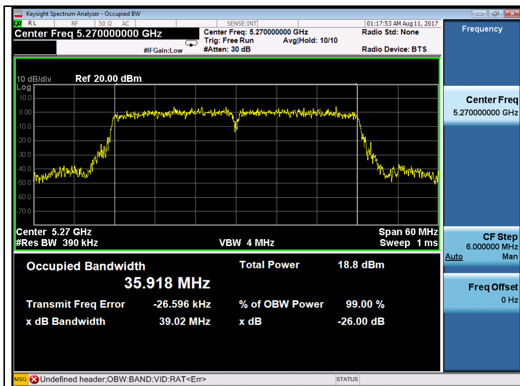
802.11n-HT40-5270MHz
