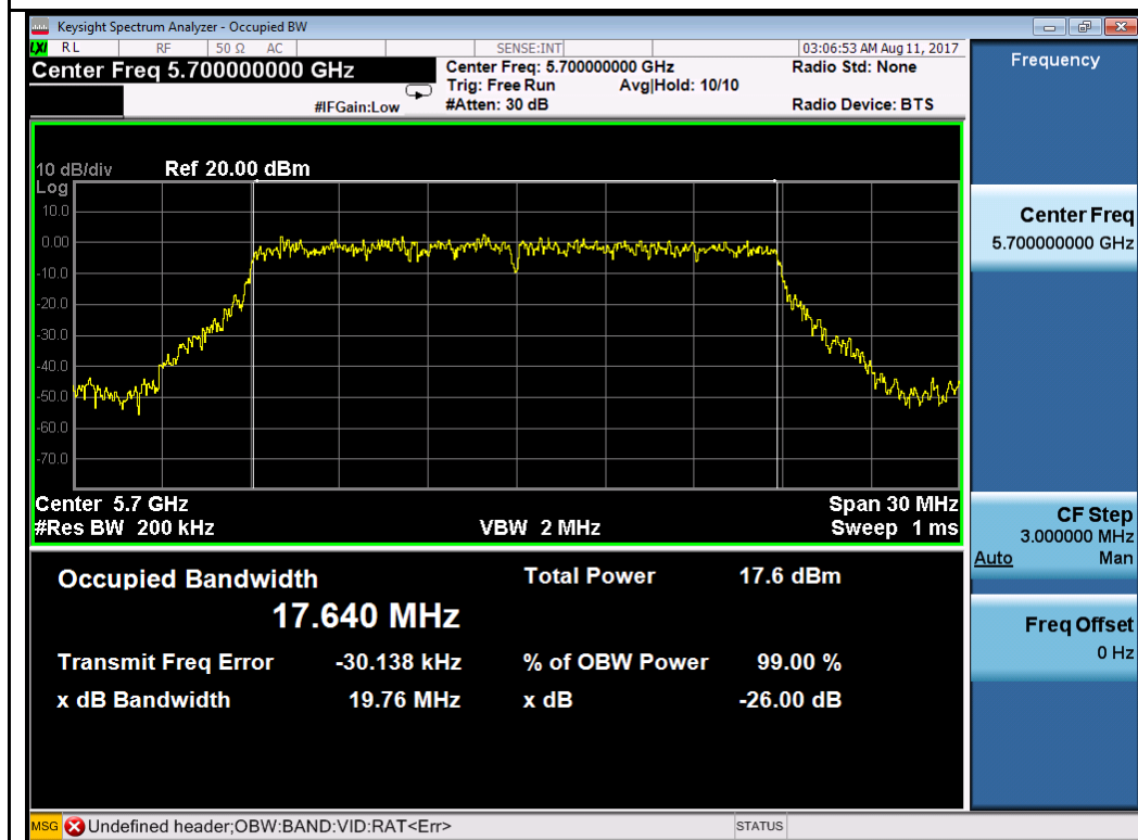
802.11n-HT20-5700MHz
