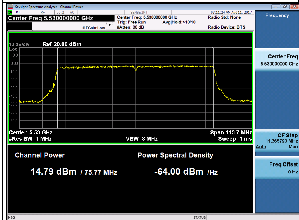
802.11ac-VHT80 5530M
