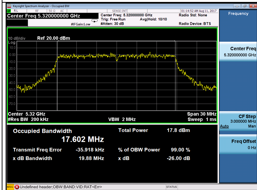
802.11n-HT20-5320MHz
