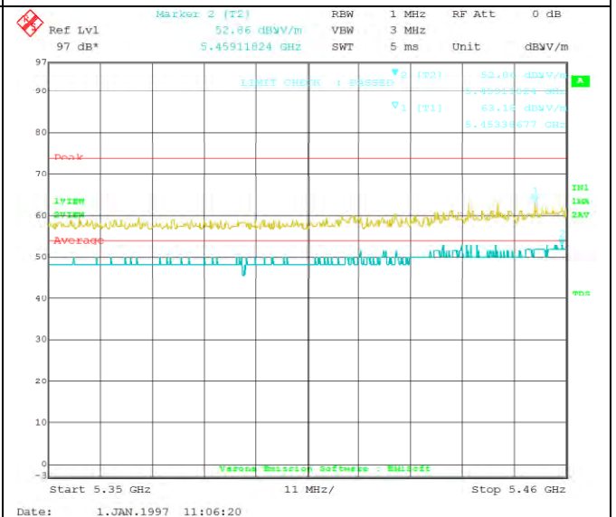
802.11ac 5530M(5350-5460MHz)
