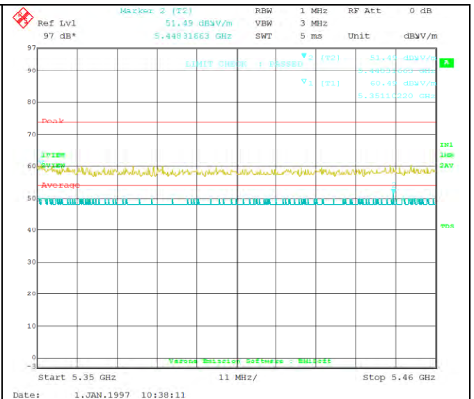
802.11n-HT20 5320M(5350-5460MHz)
