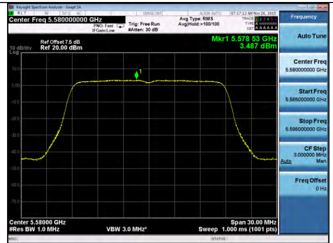
PSD-802.11n-20M-5580M-chain4
