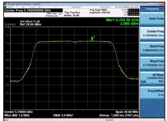
PSD-802.11n-20M-5700M-chain4
