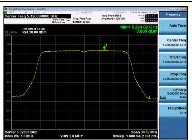
PSD-802.11n-20M-5320M-chain2
