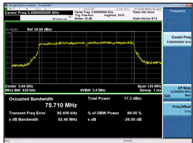
26dB BW -802.11ac CROSS 5690MHz
