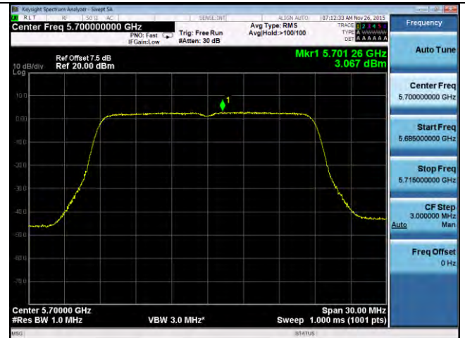
PSD-802.11n-20M-5700M-chain2
