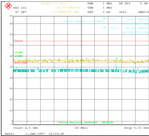
802.11a 5180M
