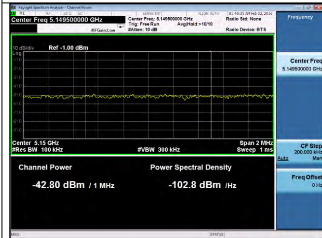
Band Edge -802.11a-5180M-chain3
