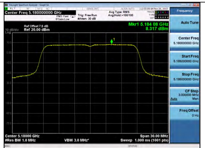
PSD-802.11n-20M-5180M-chain4
