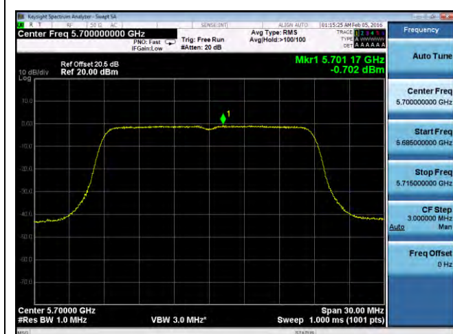
PSD-802.11n-20M-5700M-chain3
