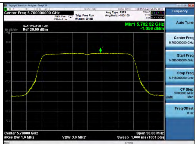
PSD-802.11n-20M-5700M-chain2
