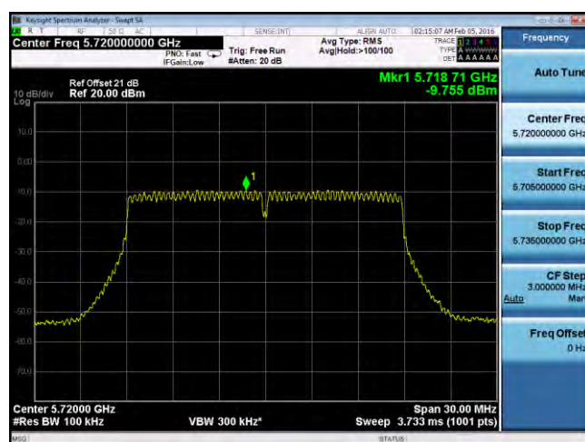
PSD-802.11n-20M-CROSS-5720M-chain4
