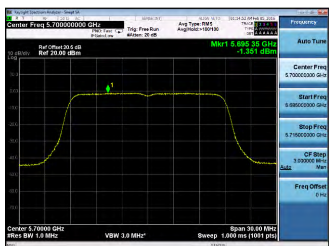
PSD-802.11n-20M-5700M-chain4
