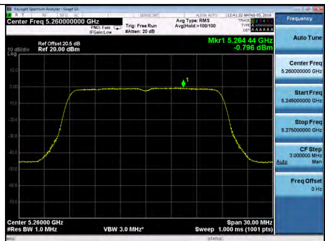
PSD-802.11n-20M-5260M-chain4
