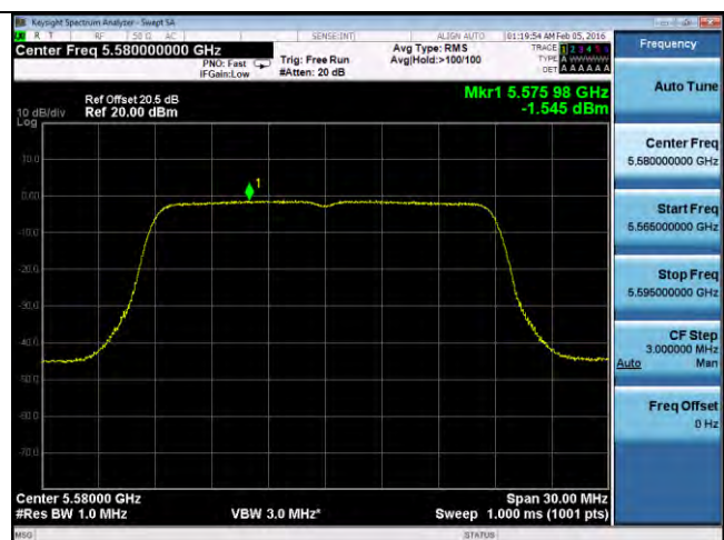
PSD-802.11n-20M-5580M-chain4
