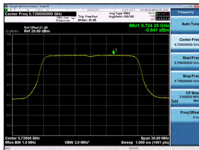
PSD-802.11n-20M-CROSS-5720M-chain4
