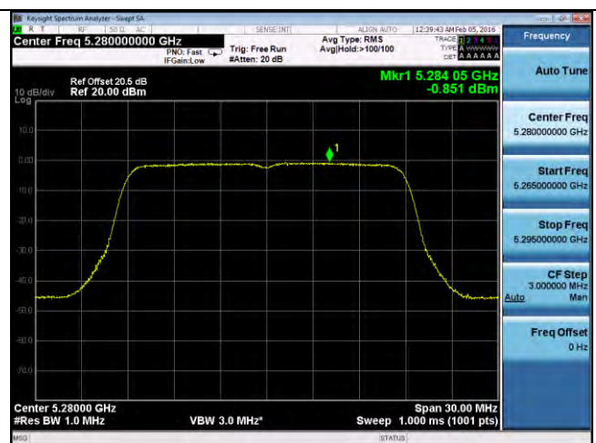
PSD-802.11n-20M-5280M-chain4
