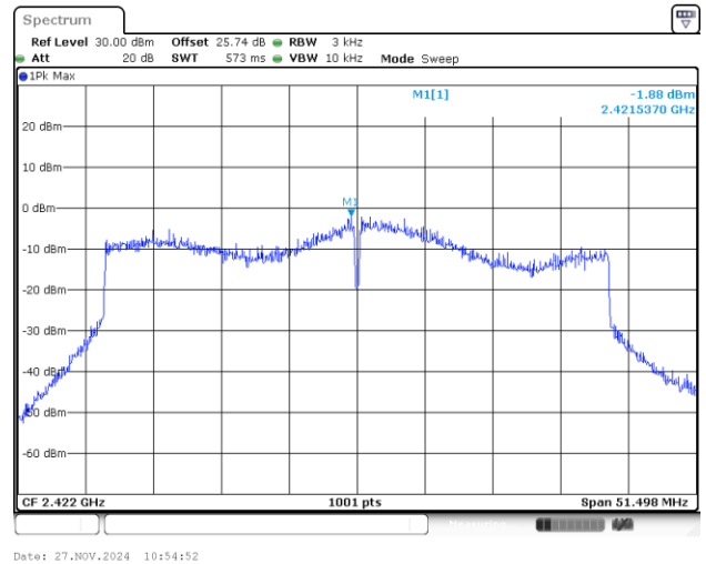
MIMO Ant 3
