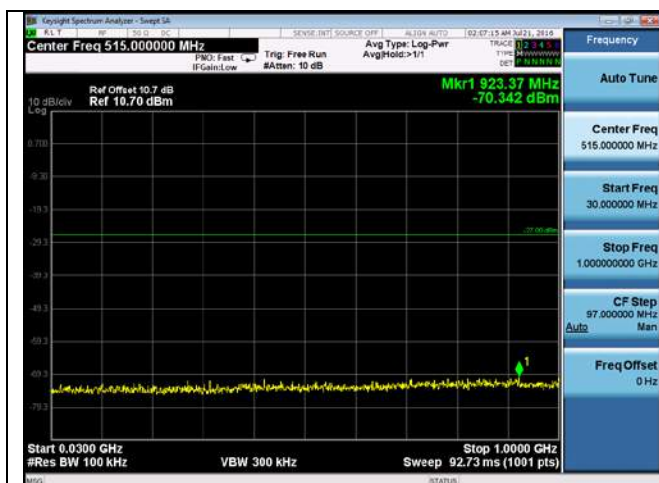
CUE-802.11n20-5720M -chain4(30MHz-1GHz)
