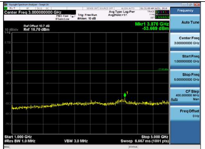
CUE-802.11n40-5710M -chain3(1GHz-5GHz)
