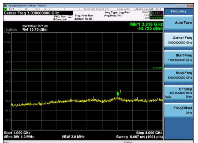
CUE-802.11n40-5710M -chain4(1GHz-5GHz)
