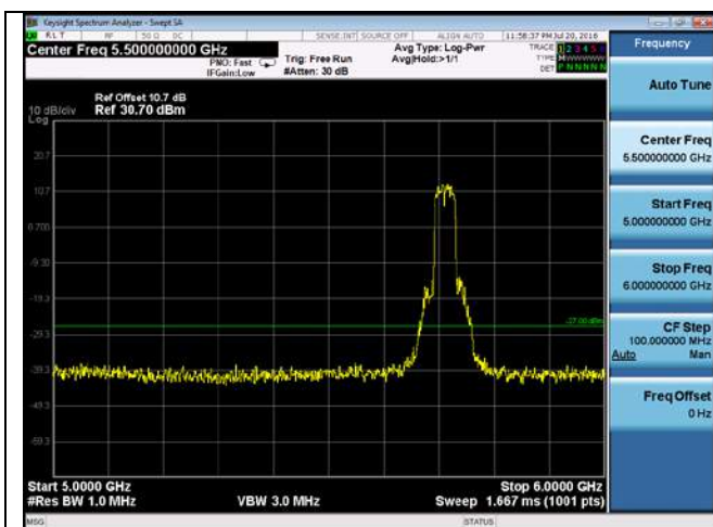
CUE-802.11n40-5710M -chain1 (5GHz-6GHz)
