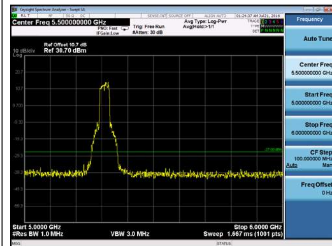
CUE-802.11n-40-5270M-chain3(5GHz-6GHz)
