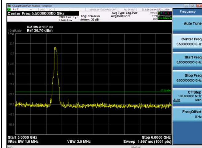
CUE-802.11a-5260-chain3(5GHz-6GHz)
