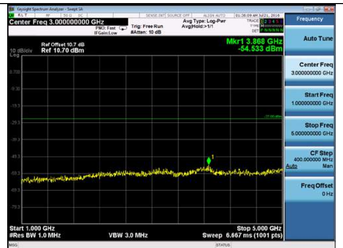
CUE-802.11ac-80-5530M -chain3(1GHz-5GHz)
