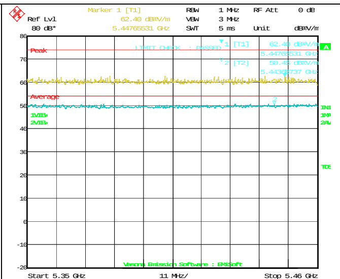
802.11n-HT20 5320M(5350-5460MHz)
