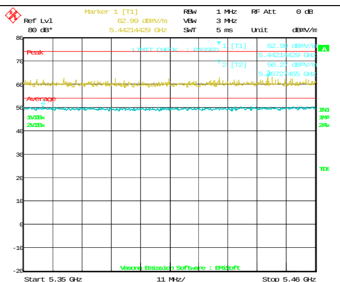
802.11n-HT20 5500M(5350-5460MHz)
