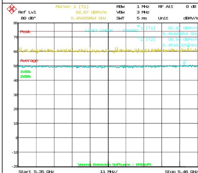
802.11n-HT40 5310M(5350-5460MHz)
