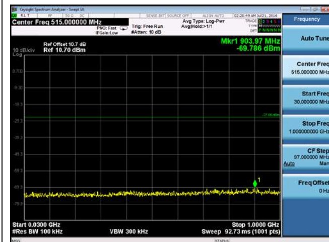
CUE-802.11ac-80-5610M-chain4(30MHz-1GHz)
