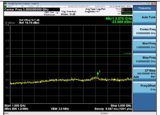
CUE-802.11n40-5710M -chain3(1GHz-5GHz)
