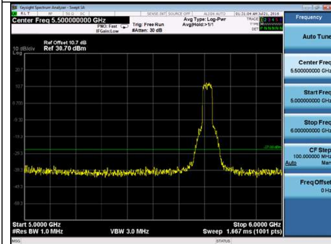
CUE-802.11n40-5710M -chain3(5GHz-6GHz)
