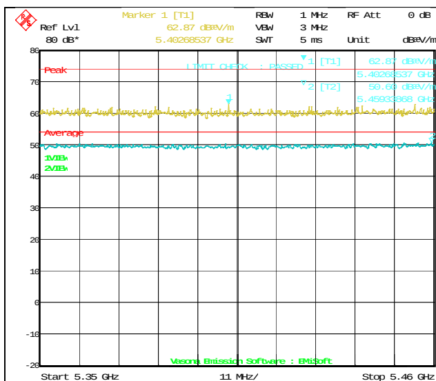
802.11a 5500M(5350-5460MHz)
