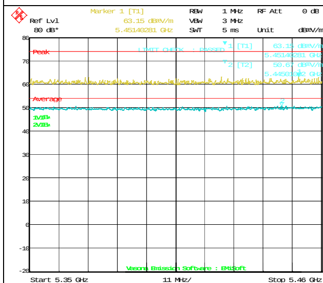
802.11n-HT40 5510M(5350-5460MHz)
