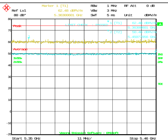
802.11ac 5530M(5350-5460MHz)
