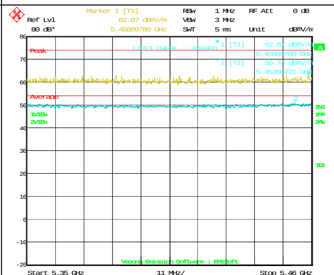
802.11ac 5290M(5350-5460MHz)
