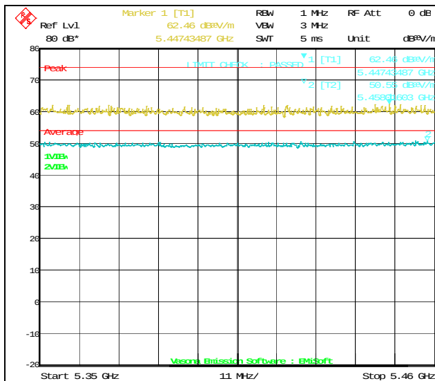
802.11a 5320M(5350-5460MHz)
