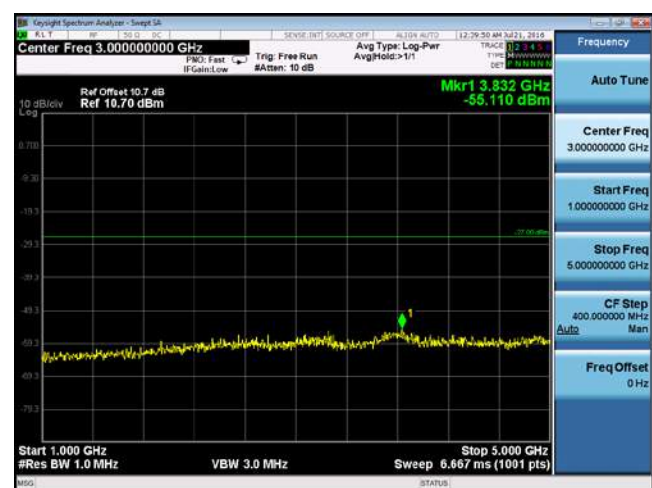
CUE-802.11n40-5710M -chain2 (1GHz-5GHz)
