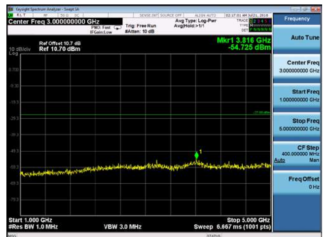
CUE-802.11n40-5710M -chain4(1GHz-5GHz)
