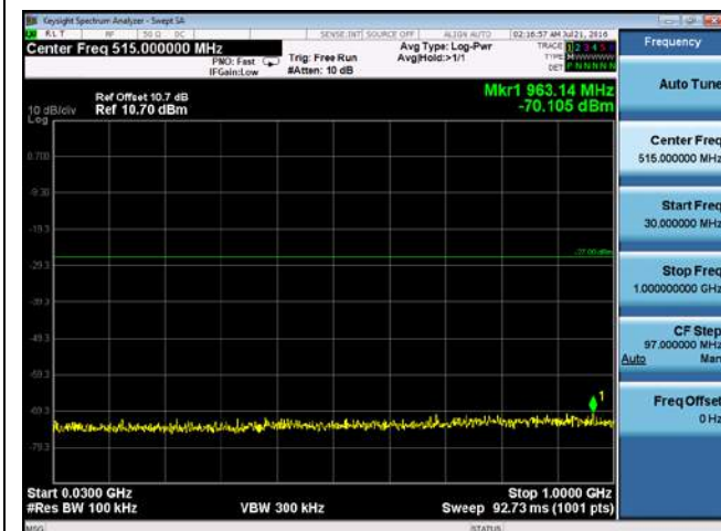
CUE-802.11n40-5710M -chain4(30MHz-1GHz)
