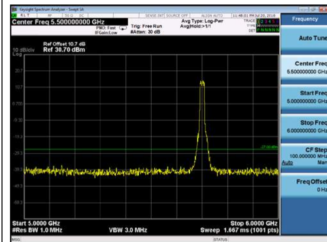
CUE-802.11n-20-5700M -chain 1(5GHz-6GHz)
