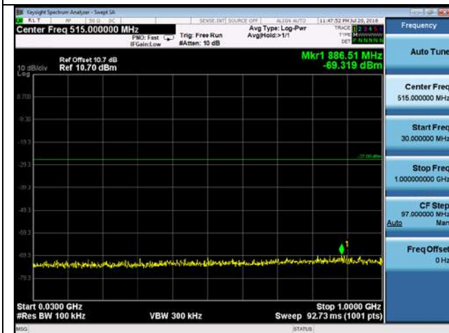
CUE-802.11n-20-5700M -chain 1(30MHz-1GHz)
