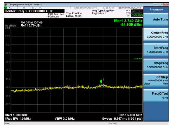
CUE-802.11n-20-5700M -chain 1(1GHz-5GHz)
