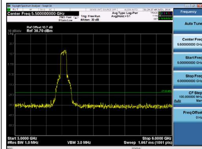
CUE-802.11n-40-5270M-chain3(5GHz-6GHz)
