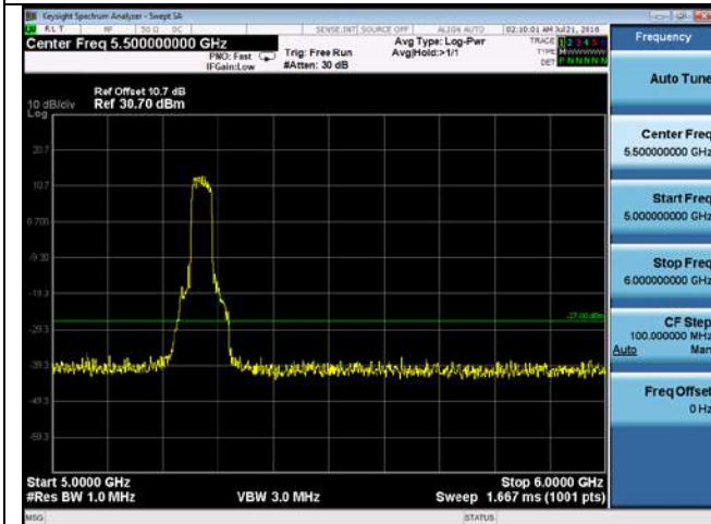
CUE-802.11n-40-5270M-chain4(5GHz-6GHz)
