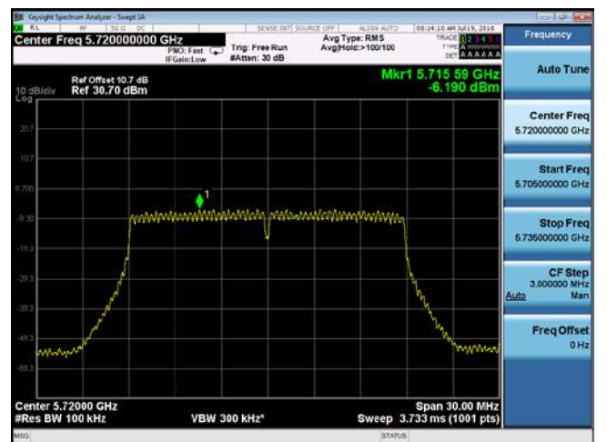
PSD-802.11n-20M-CROSS-5720M-chain4
