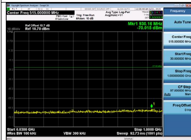
CUE-802.11ac-80-5775M-chain 1(30MHz-1GHz)
