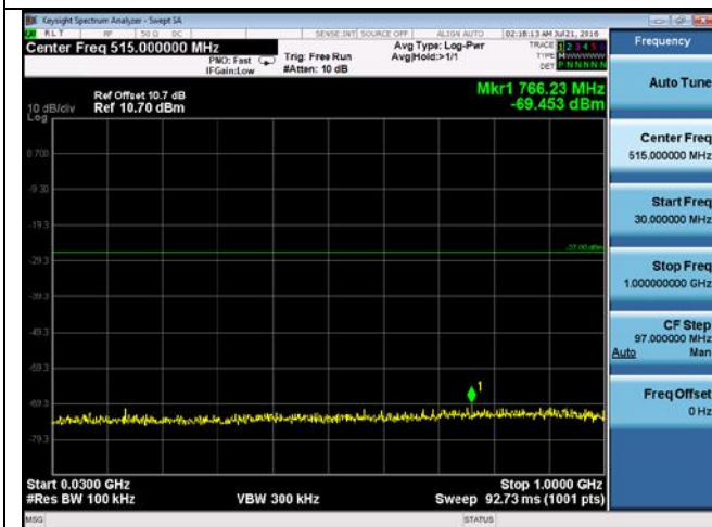
CUE-802.11ac-80-5210M -chain 4(30MHz-1GHz)
