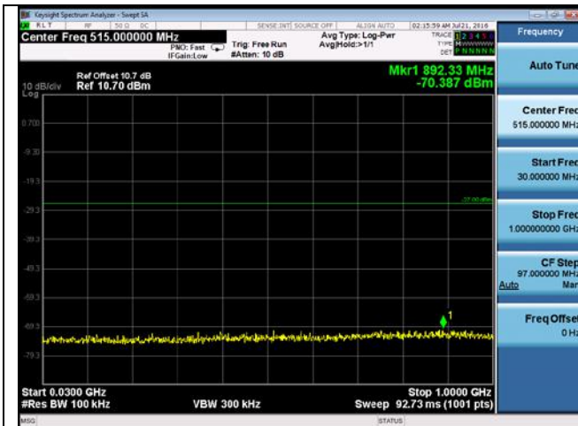
CUE-802.11n-40-5755M-chain4(30MHz-1GHz)
