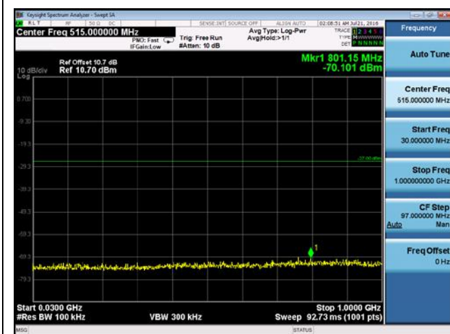
CUE-802.11n-40-5230M -chain4(30MHz-1GHz)
