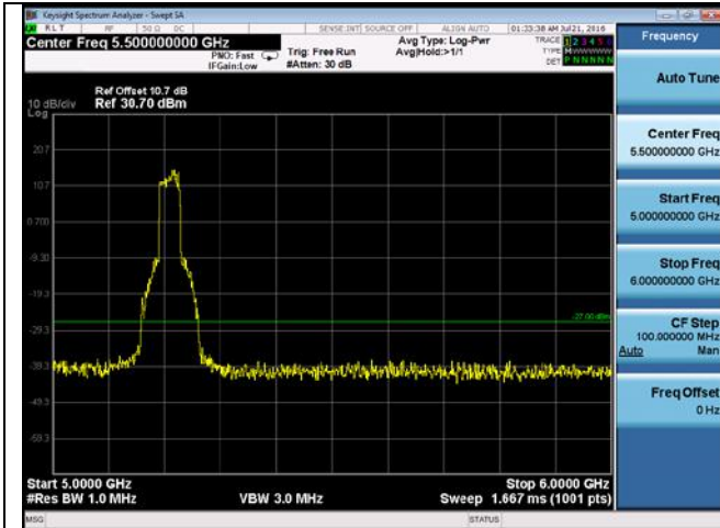
CUE-802.11ac-80-5210M -chain 3(5GHz-6GHz)
