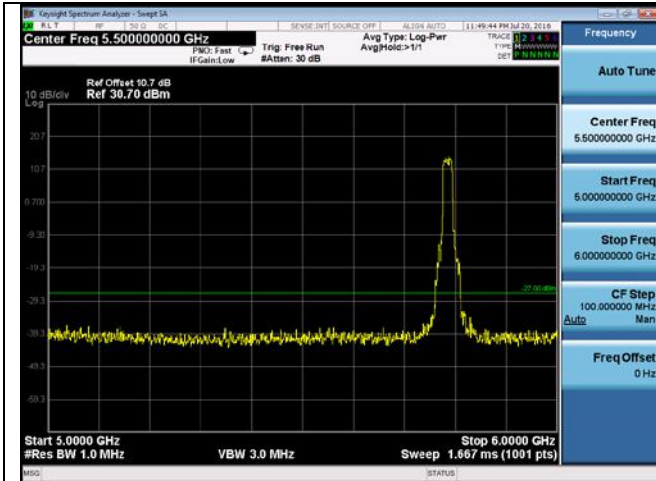
CUE-802.11n-20-5785M -chain1(5GHz-6GHz)
