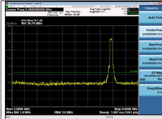
CUE-802.11n-20-5785M -chain 4(5GHz-6GHz)
