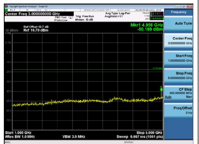
CUE-802.11n-40-5230M -chain4(1GHz-5GHz)
