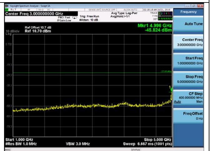
CUE-802.11ac-80-5210M -chain 4(1GHz-5GHz)
