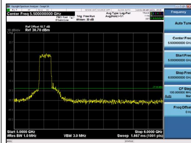
CUE-802.11ac-80-5210M-chain 1(5GHz-6GHz)
