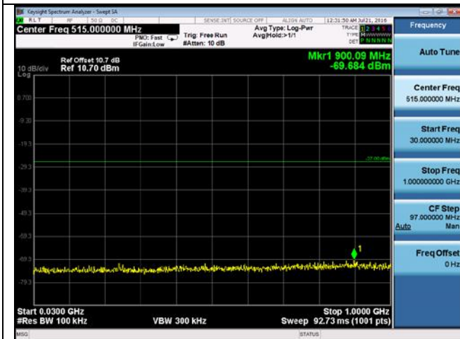
CUE-802.11n-40-5230M -chain2(30MHz-1GHz)
