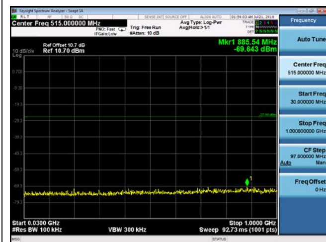
CUE-802.11a-5785M-chain4(30MHz-1GHz)
