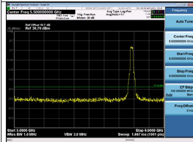
CUE-802.11n-20-5785M -chain3(5GHz-6GHz)
