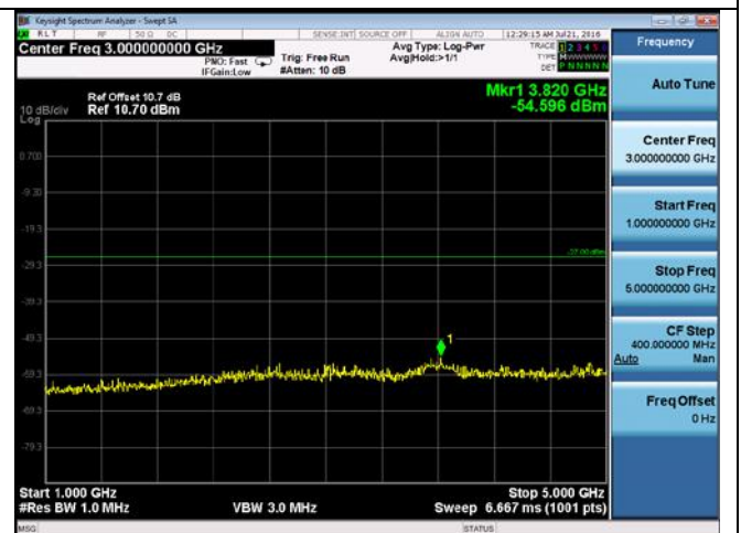
CUE-802.11n-20-5785M -chain2(1GHz-5GHz)
