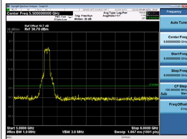
CUE-802.11n-40-5230M -chain2(5GHz-6GHz)
