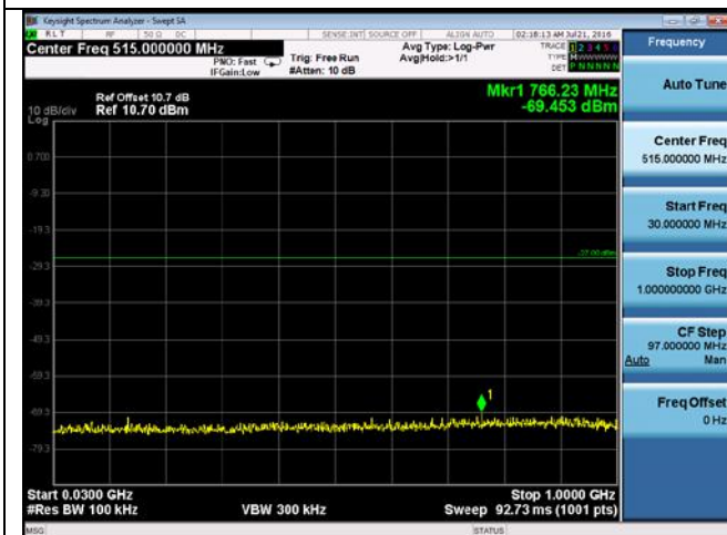
CUE-802.11ac-80-5210M -chain 4(30MHz-1GHz)
