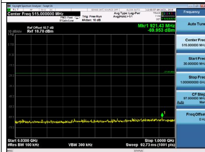
CUE-802.11ac-80-5210M-chain 1(30MHz-1GHz)
