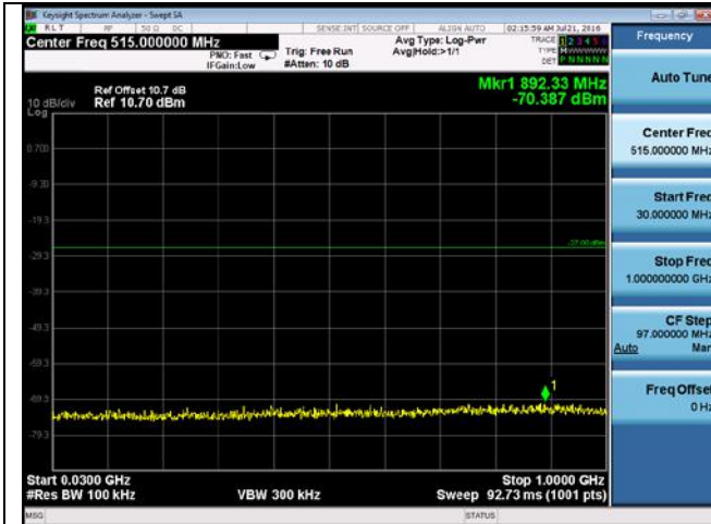
CUE-802.11n-40-5755M-chain4(30MHz-1GHz)
