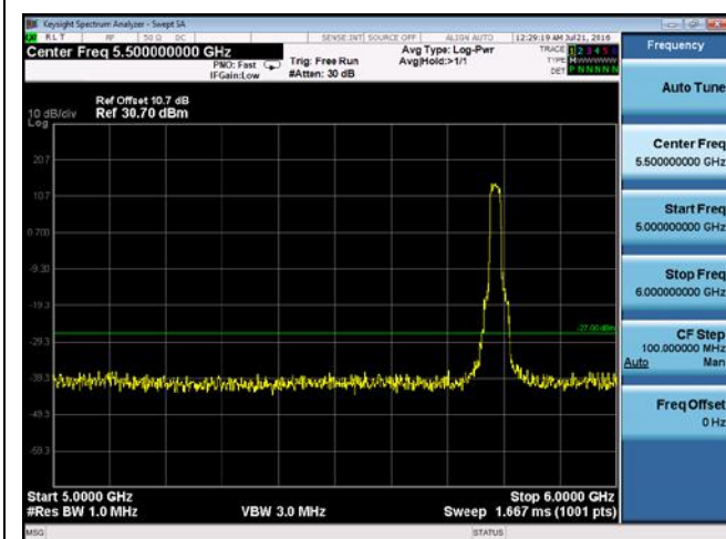
CUE-802.11n-20-5785M -chain2(5GHz-6GHz)
