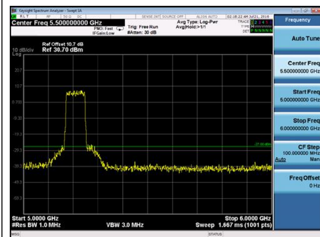
CUE-802.11ac-80-5210M -chain 4(5GHz-6GHz)
