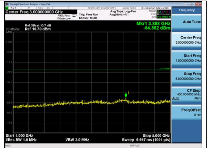
CUE-802.11n-20-5785M -chain3(1GHz-5GHz)
