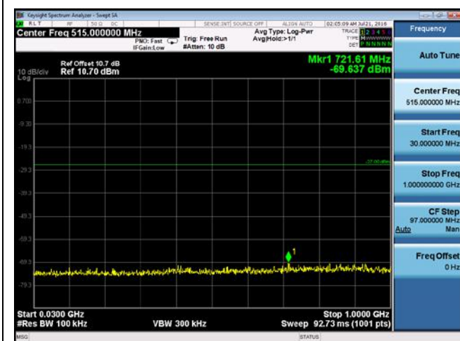
CUE-802.11n-20-5785M -chain4(30MHz-1GHz)
