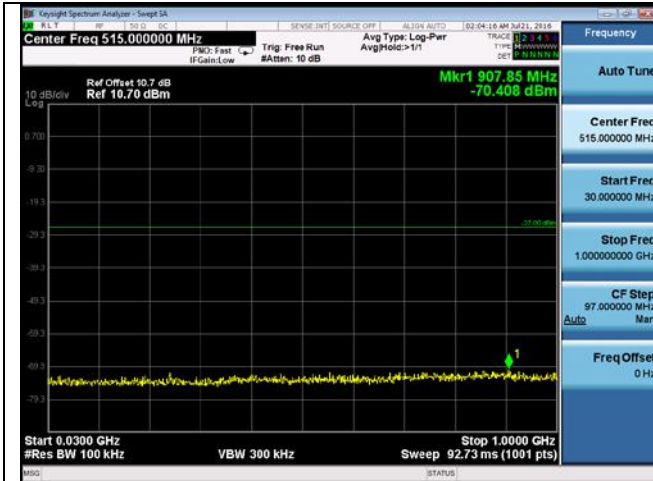
CUE-802.11n-20-5745M-chain4(30MHz-1GHz)
