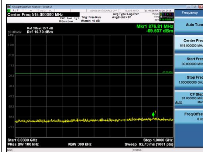
CUE-802.11n-20-5785M-chain1(30MHz-1GHz)
