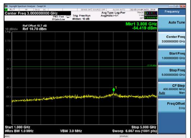
CUE-802.11n-20-5785M -chain4(1GHz-5GHz)
