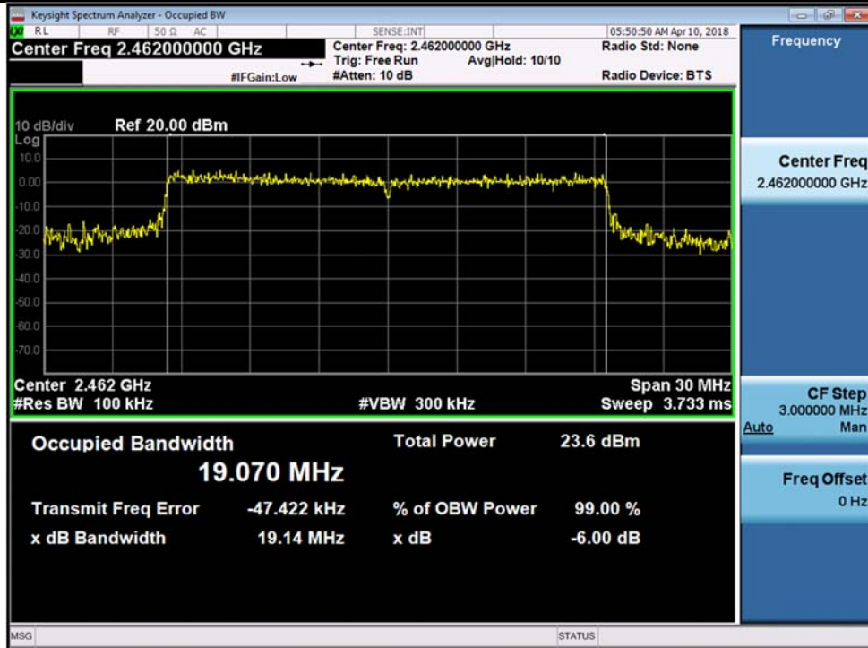
802.11ax20-2462MHz
