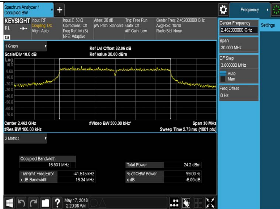
802.11g-2462MHz
