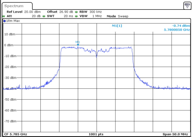
MIMO Ant. 4
