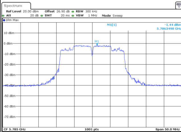
MIMO Ant. 3
