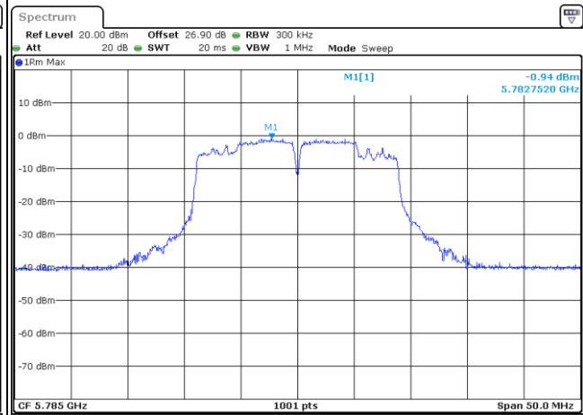
MIMO Ant. 2
