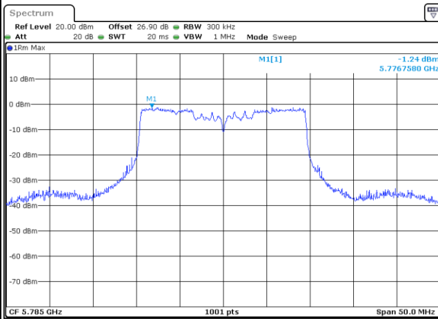
MIMO Ant. 1
