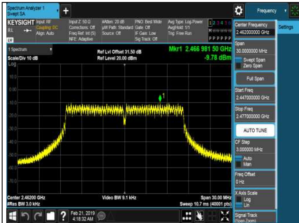
802.11g-2462MHz Chain 2
