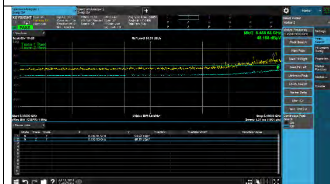
802.11ax40 5510M(5350-5460MHz)
