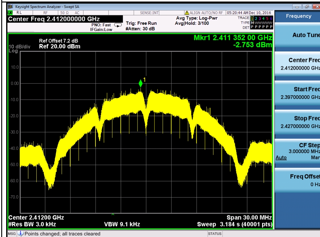
802.11b-2412MHz Chain 2
