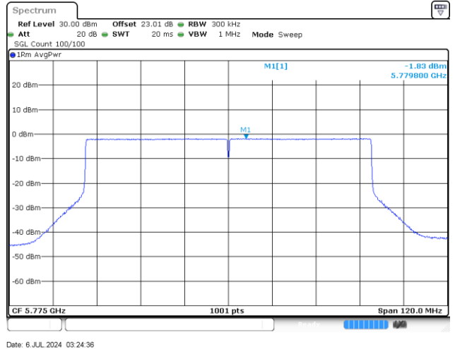
MIMO Ant. 2
