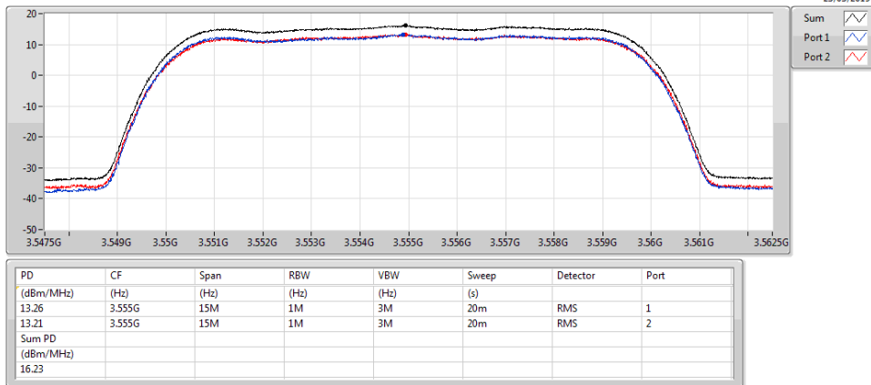
Band 48_LTE_10MHz_Nss1,QPSK_2TX 3555MHz_QPSK_RB 50,#RB 0
