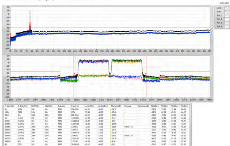
Band 48_LTE_20MHz+20MHz_Nss1,64QAM_4TX P#3670MHz,#3690MHz 64QAM RB 100,#RB 0+RB 100,#RB 0
