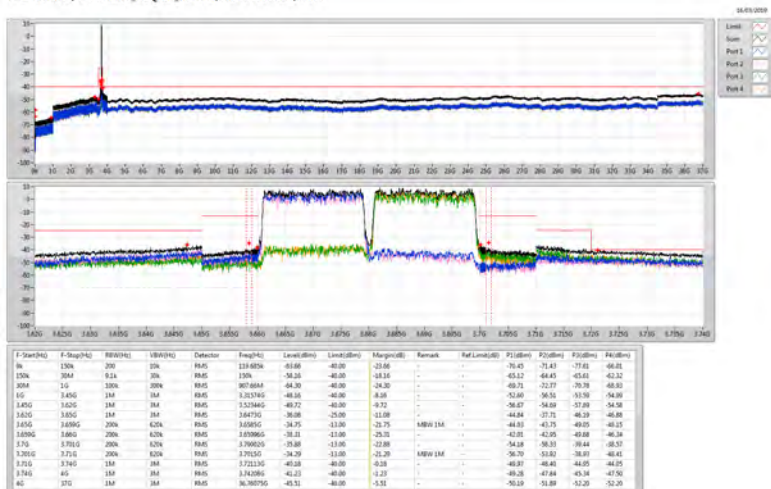
Band 48_LTE_20MHz+20MHz_Nss1,16QAM_4TX P#3560MHz,#3690MHz 16QAM RB 100,#RB 0+RB 100,#RB 0
