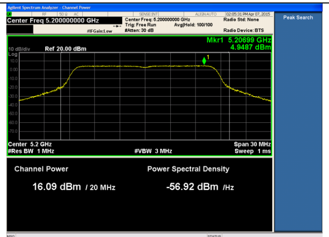
14dB ANT-PSD-802.11a-5200M-chain2
