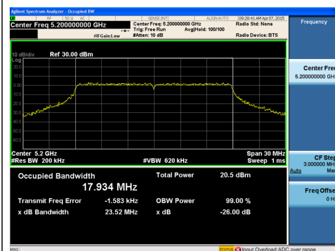
26dB BW - 802.11n-HT20 5200MHz
