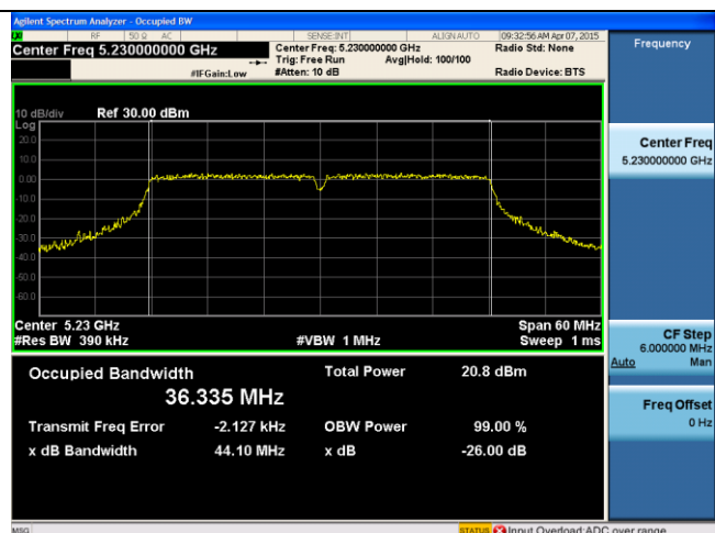
26dB BW - 802.11n-HT40 5230MHz
