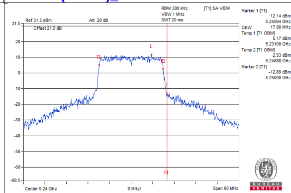
802.11ac(VHT20)_Chain1 / CH48
