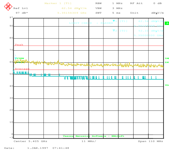
802.11ac-VHT80 5290M(5350-5460MHz)
