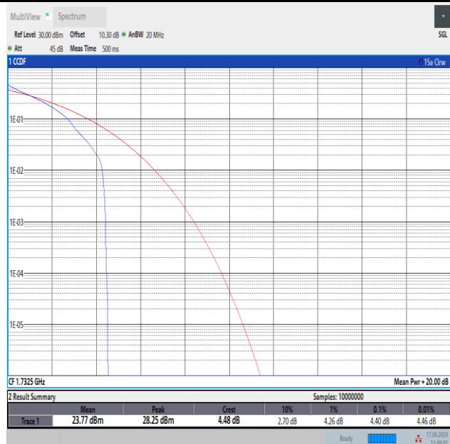
Band4-20MHz-QPSK-20175-1RB#0-PASS
