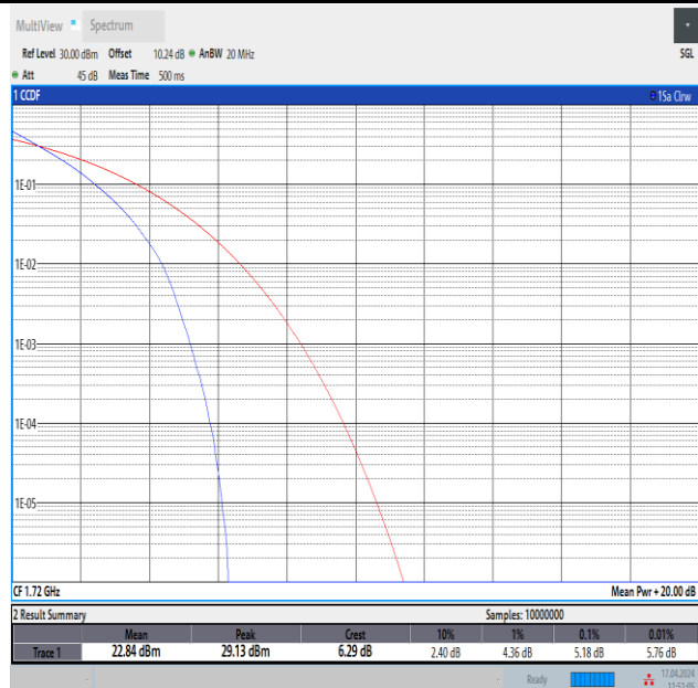
Band4-20MHz-QPSK-20050-100RB#0-PASS
