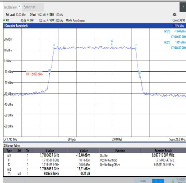
Band4-10MHz-QPSK-20000-50RB#0-PASS
