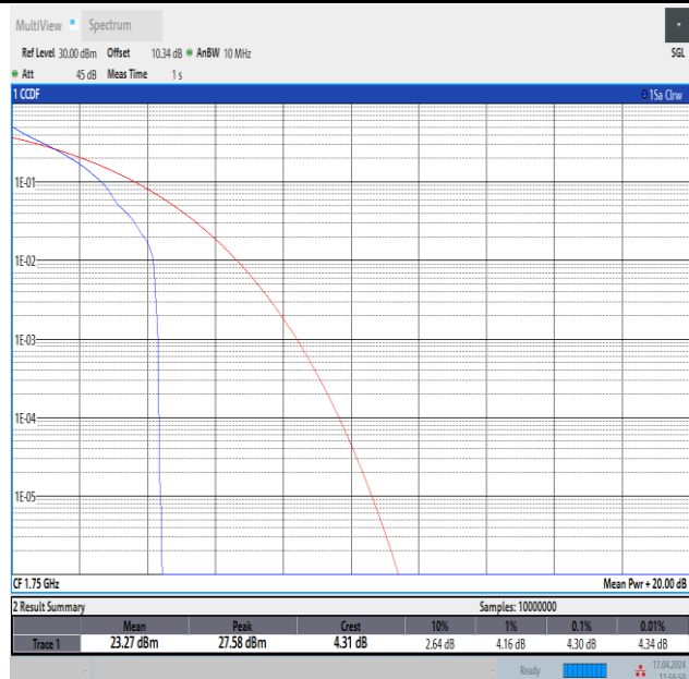
Band4-10MHz-QPSK-20350-1RB#0-PASS
