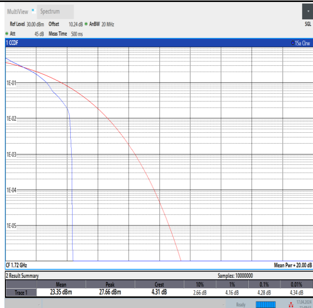
Band4-20MHz-QPSK-20050-1RB#0-PASS
