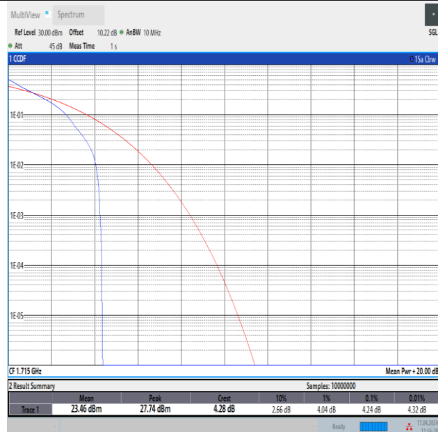
Band4-10MHz-QPSK-20000-1RB#0-PASS
