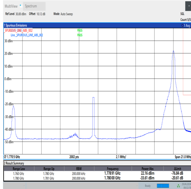
Band66_20MHz_QPSK_132572_1RB#99
