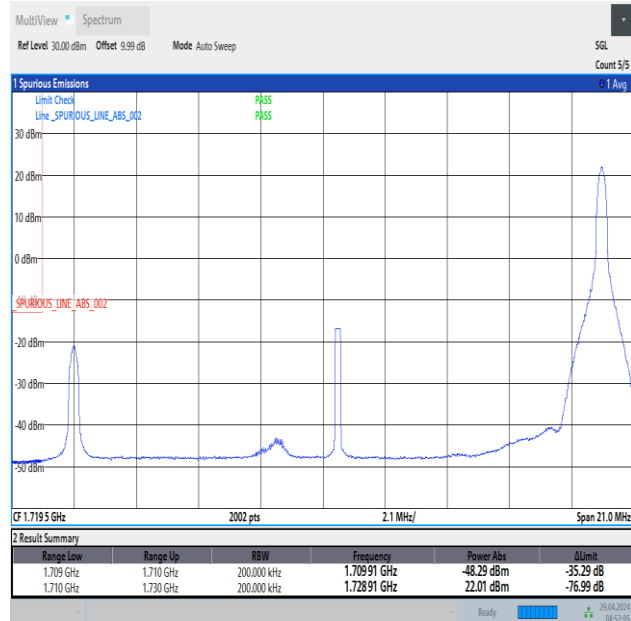
Band66_20MHz_QPSK_132072_1RB#99
