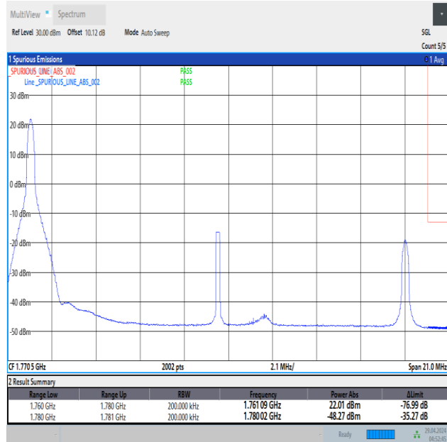
Band66_20MHz_QPSK_132572_1RB#0
