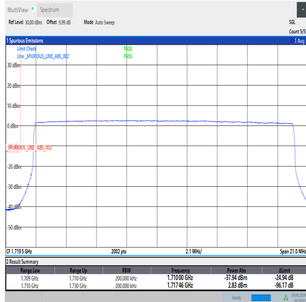
Band66_20MHz_QPSK_132072_100RB#0
