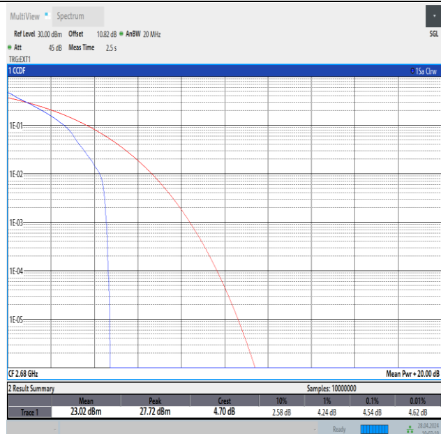
Band41-20MHz-QPSK-41490-1RB#0-PASS
