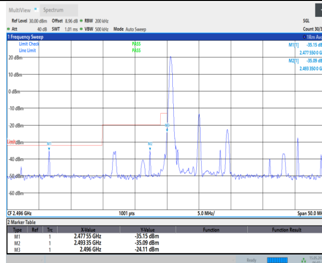
Band41-10MHz-QPSK-39700-50RB#0
