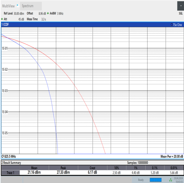
Band26(824-849)-3MHz-QPSK-26805-15RB#0-PASS
