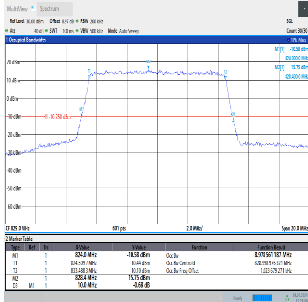
Band26(824-849)-10MHz-QPSK-26840-50RB#0-PASS
