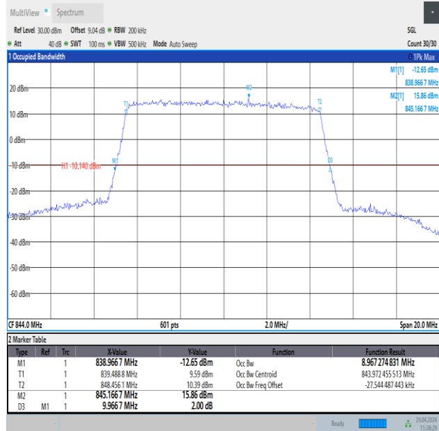
Band26(824-849)-10MHz-QPSK-26990-50RB#0-PASS
