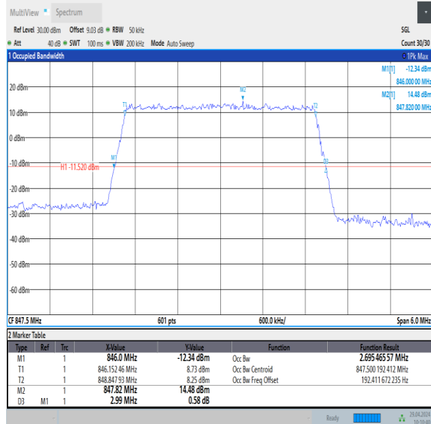
Band26(824-849)-3MHz-QPSK-27025-15RB#0-PASS
