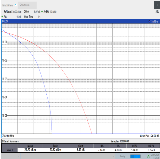
Band26(824-849)-10MHz-QPSK-26840-50RB#0-PASS
