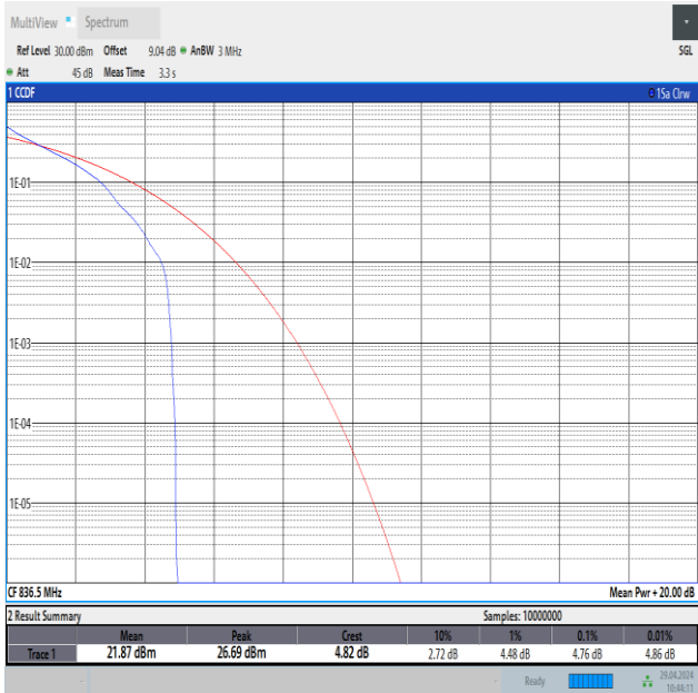
Band26(824-849)-3MHz-QPSK-26915-1RB#0-PASS
