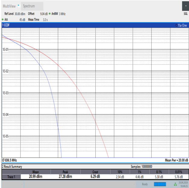
Band26(824-849)-3MHz-QPSK-26915-15RB#0-PASS
