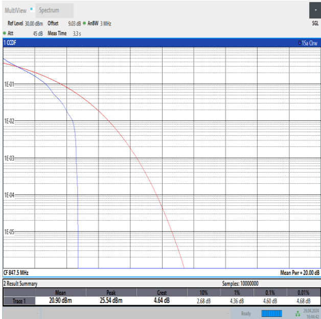
Band26(824-849)-3MHz-QPSK-27025-1RB#0-PASS
