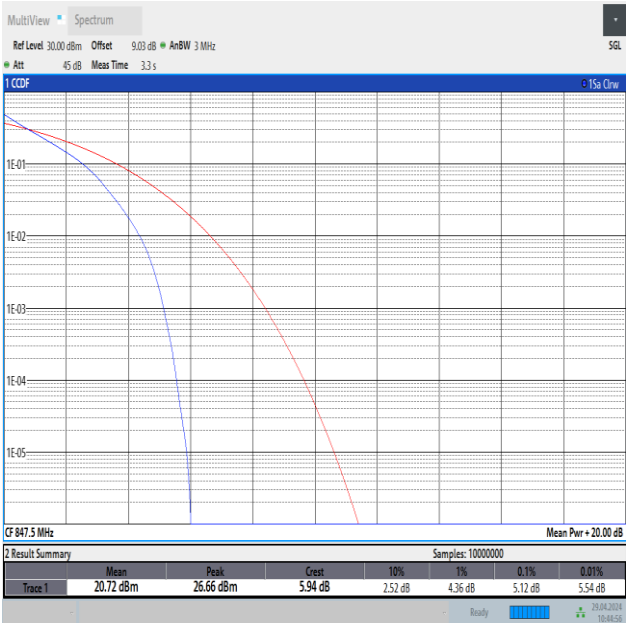
Band26(824-849)-3MHz-QPSK-27025-15RB#0-PASS
