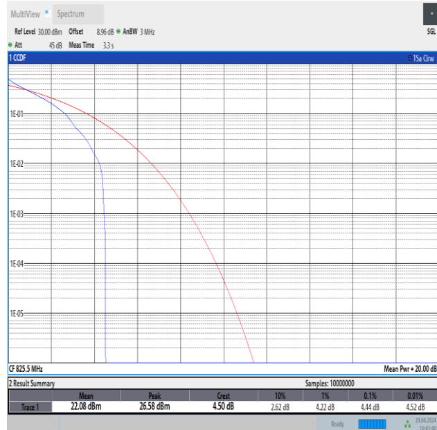
Band26(824-849)-3MHz-QPSK-26805-1RB#0-PASS
