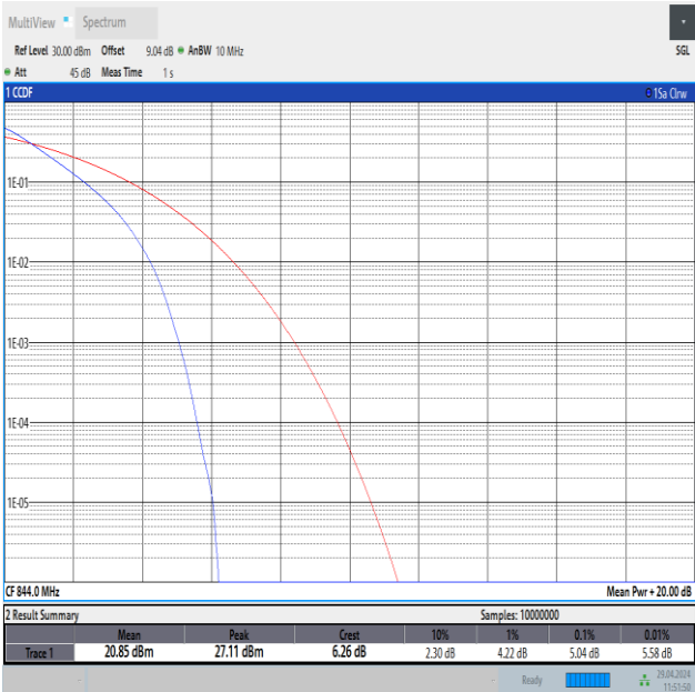
Band26(824-849)-10MHz-QPSK-26990-50RB#0-PASS
