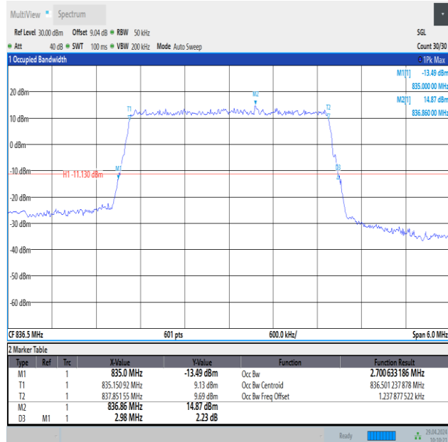
Band26(824-849)-3MHz-QPSK-26915-15RB#0-PASS
