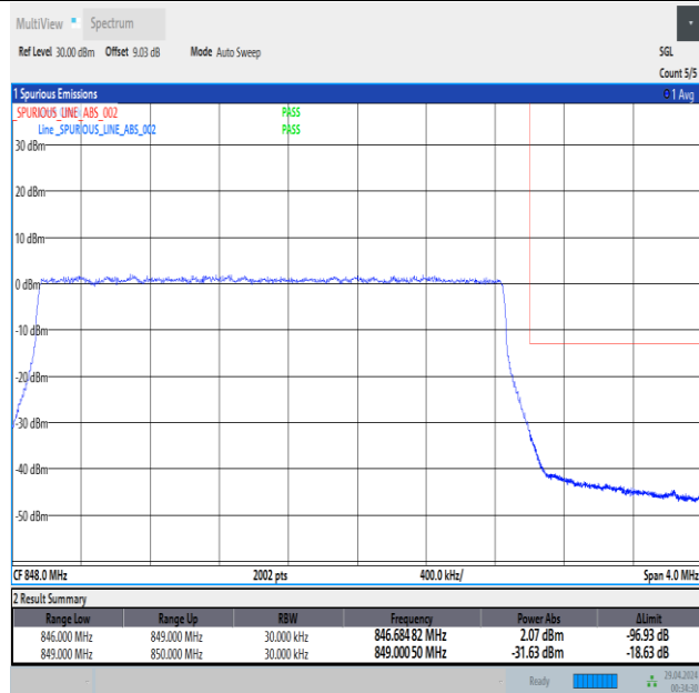
Band5_3MHz_16QAM_20635_15RB#0
