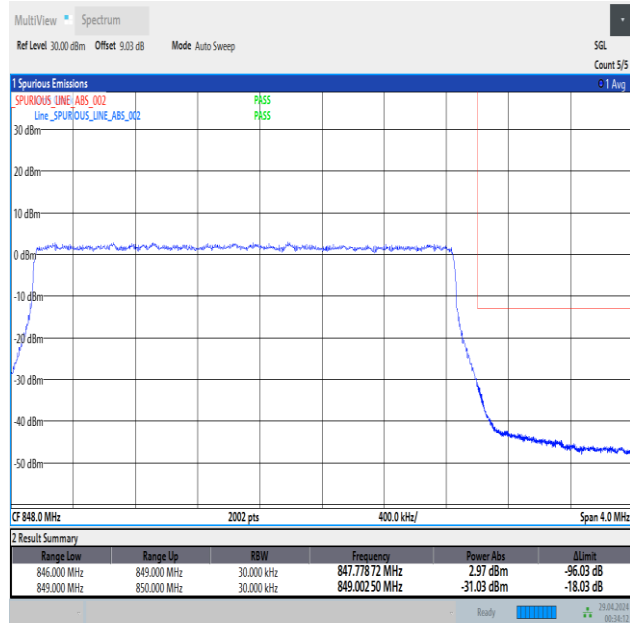
Band5_3MHz_QPSK_20635_15RB#0
