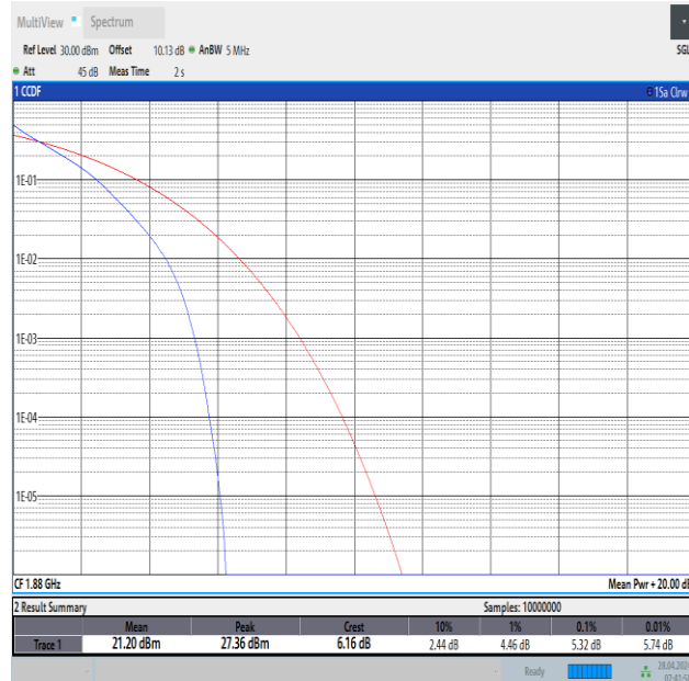
Band2-5MHz-QPSK-18900-25RB#0-PASS
