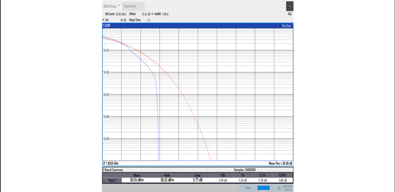
Band2-5MHz-16QAM-18625-1RB#0-PASS
