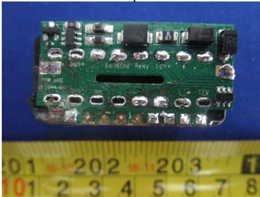
EUT – Subplate View
