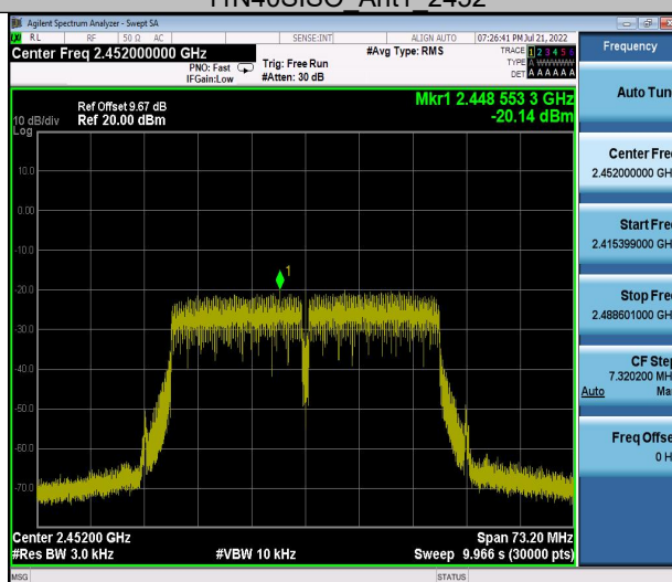
11N40SISO Ant1 2452
