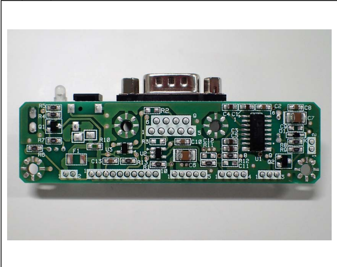
Module (I/F Unit): Bottom
