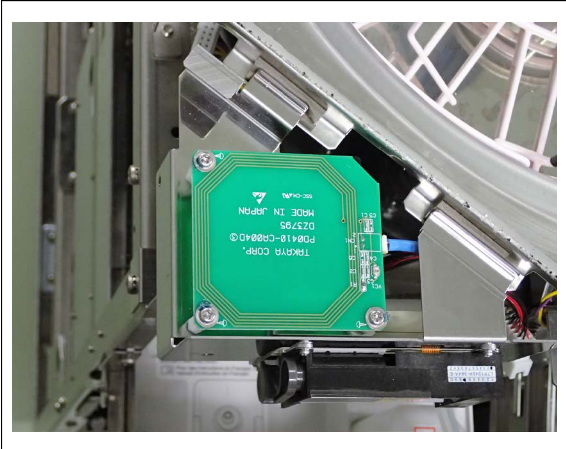
RFID Antenna
