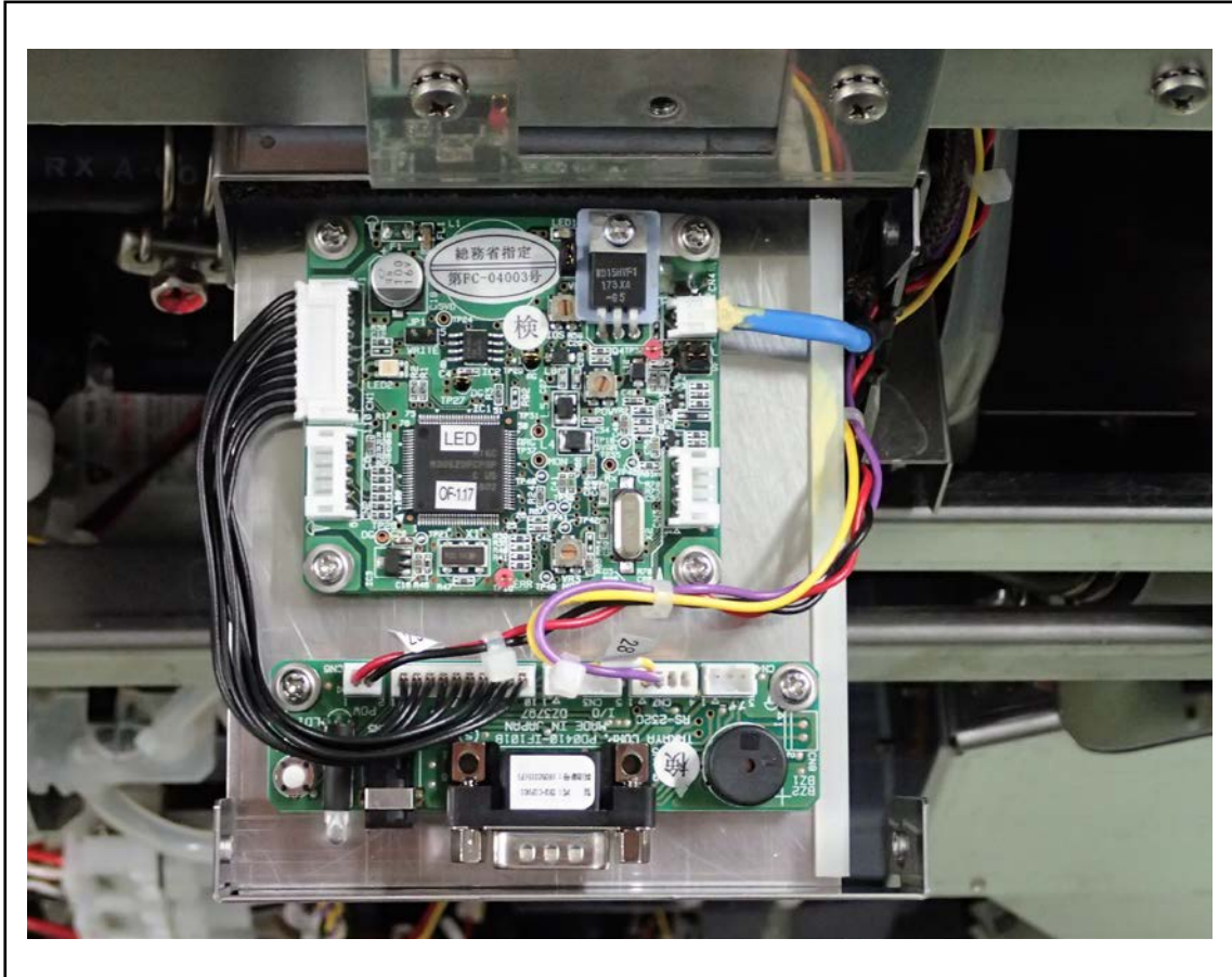
Module: R/W Unit & I/F Unit
