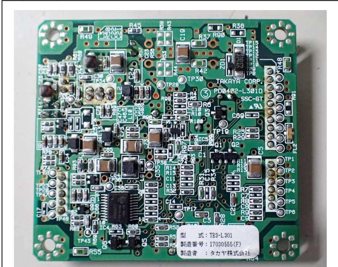
Module (R/W Unit): Bottom
