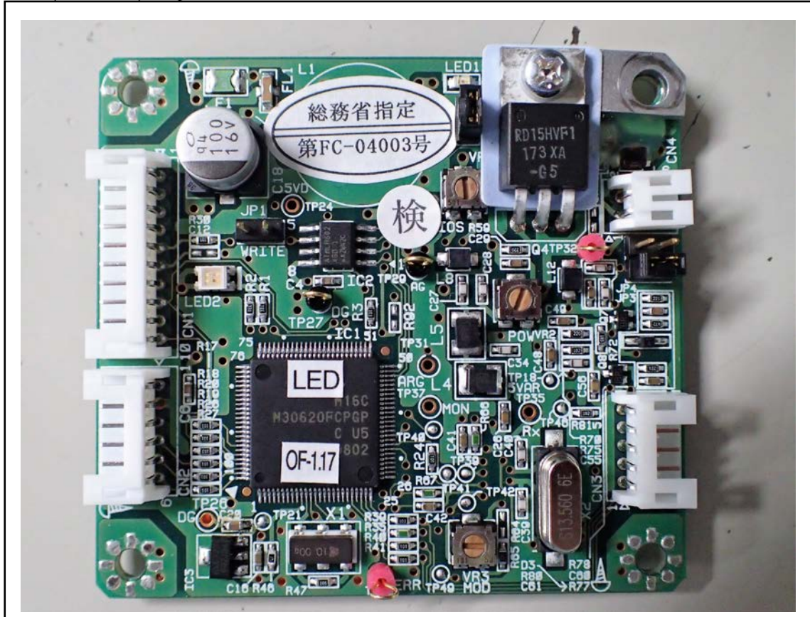
Module (R/W Unit): Top
