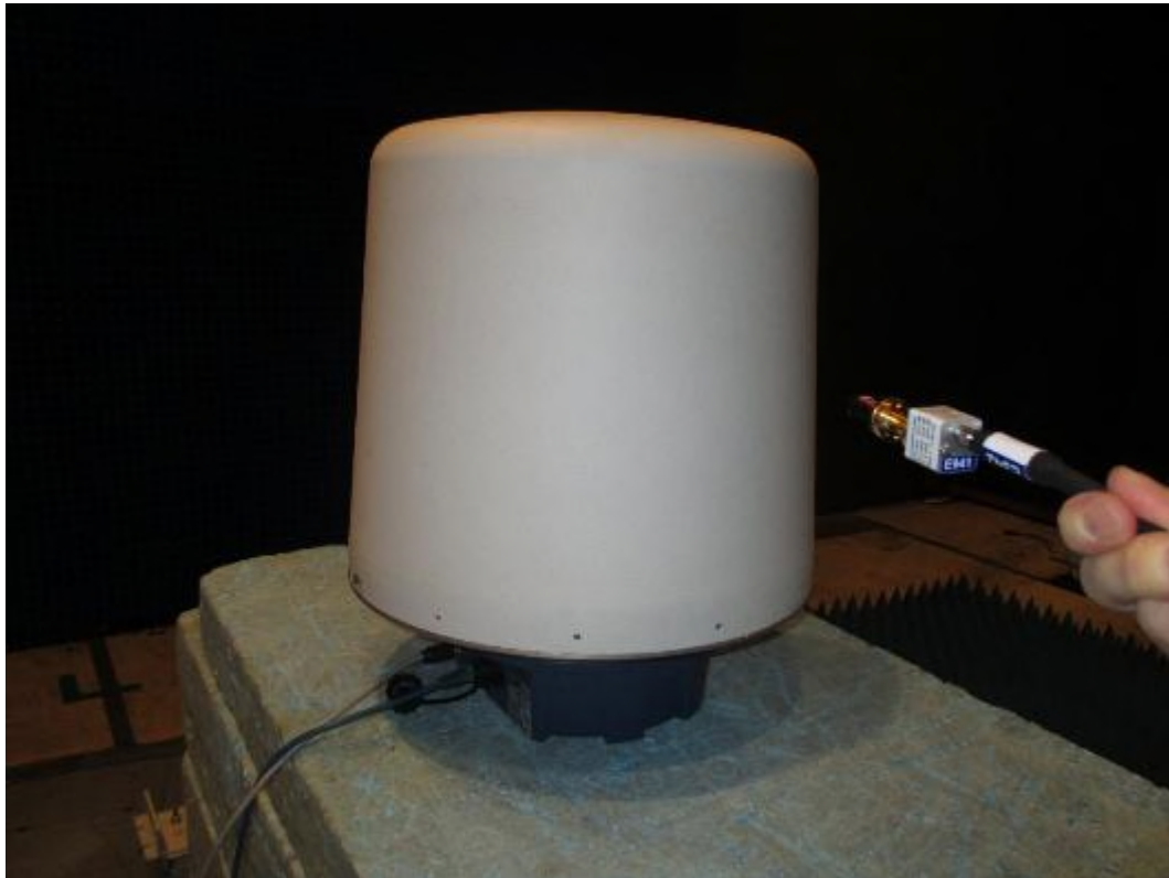
110-140 GHz
