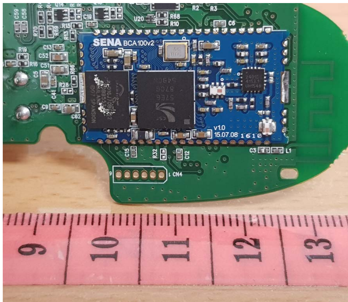
Bluetooth Module
