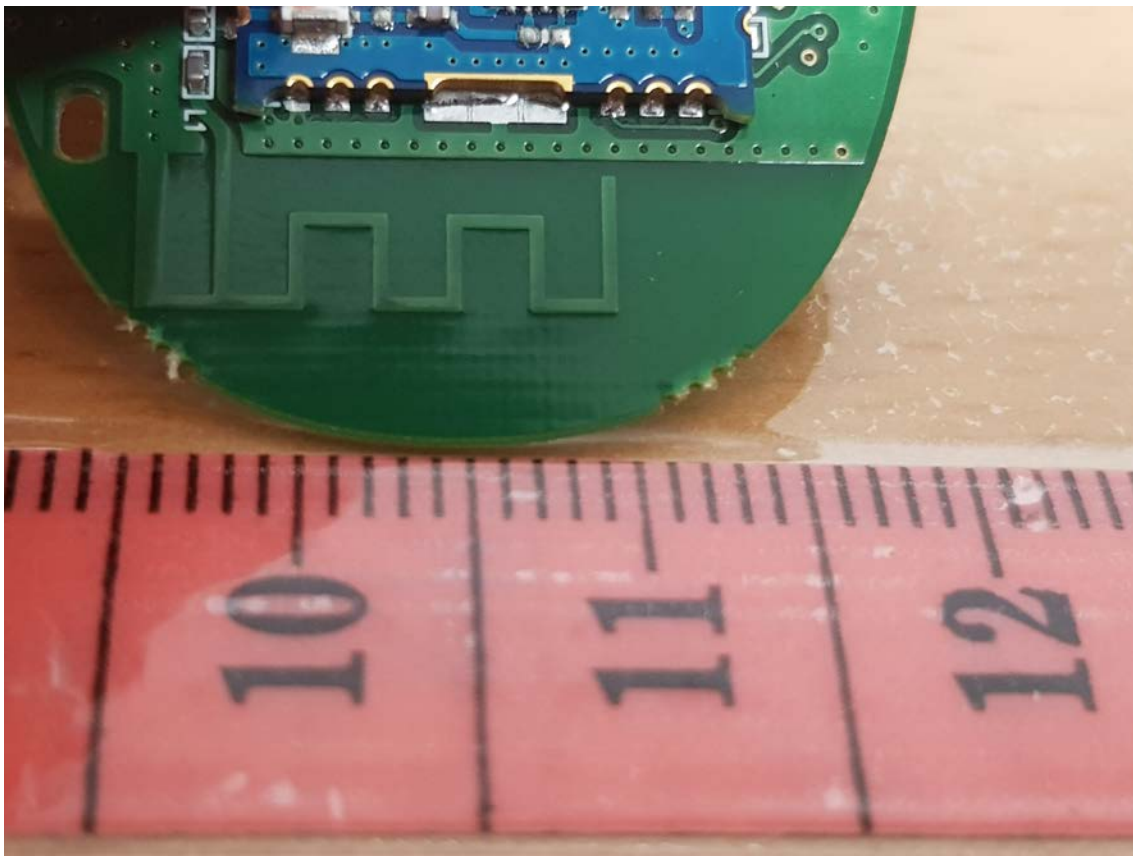
Antenna
