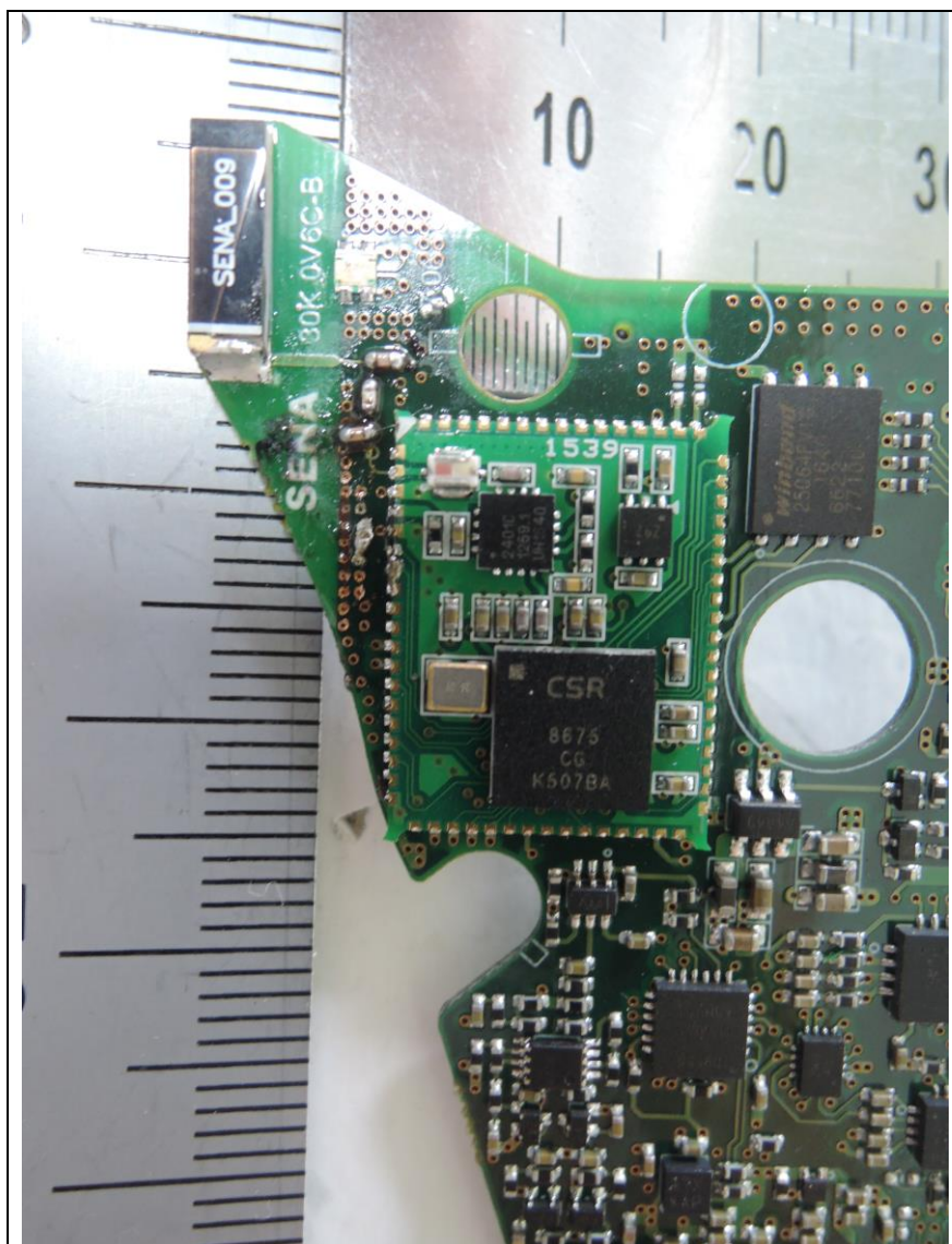
<BT Module>
