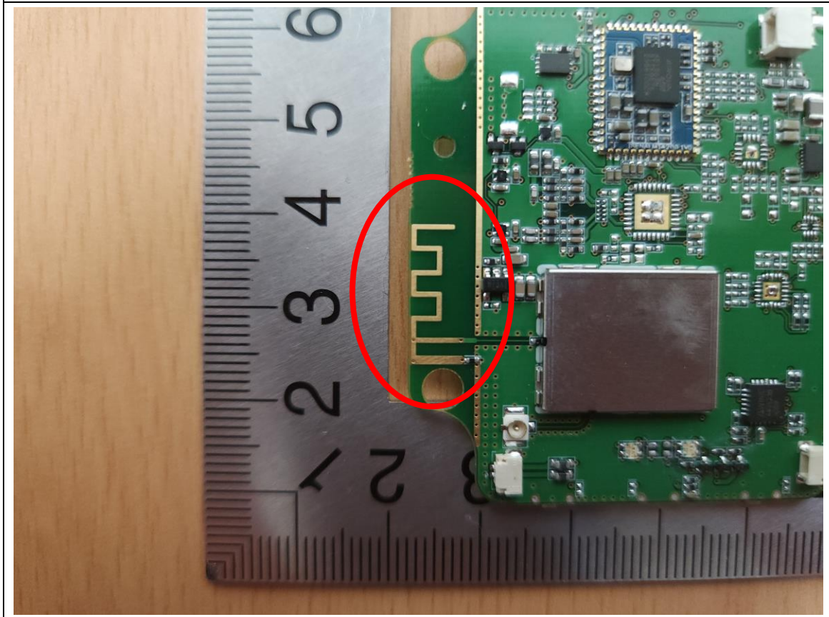
MESH Antenna 1 (M/N: Sena_P001)
